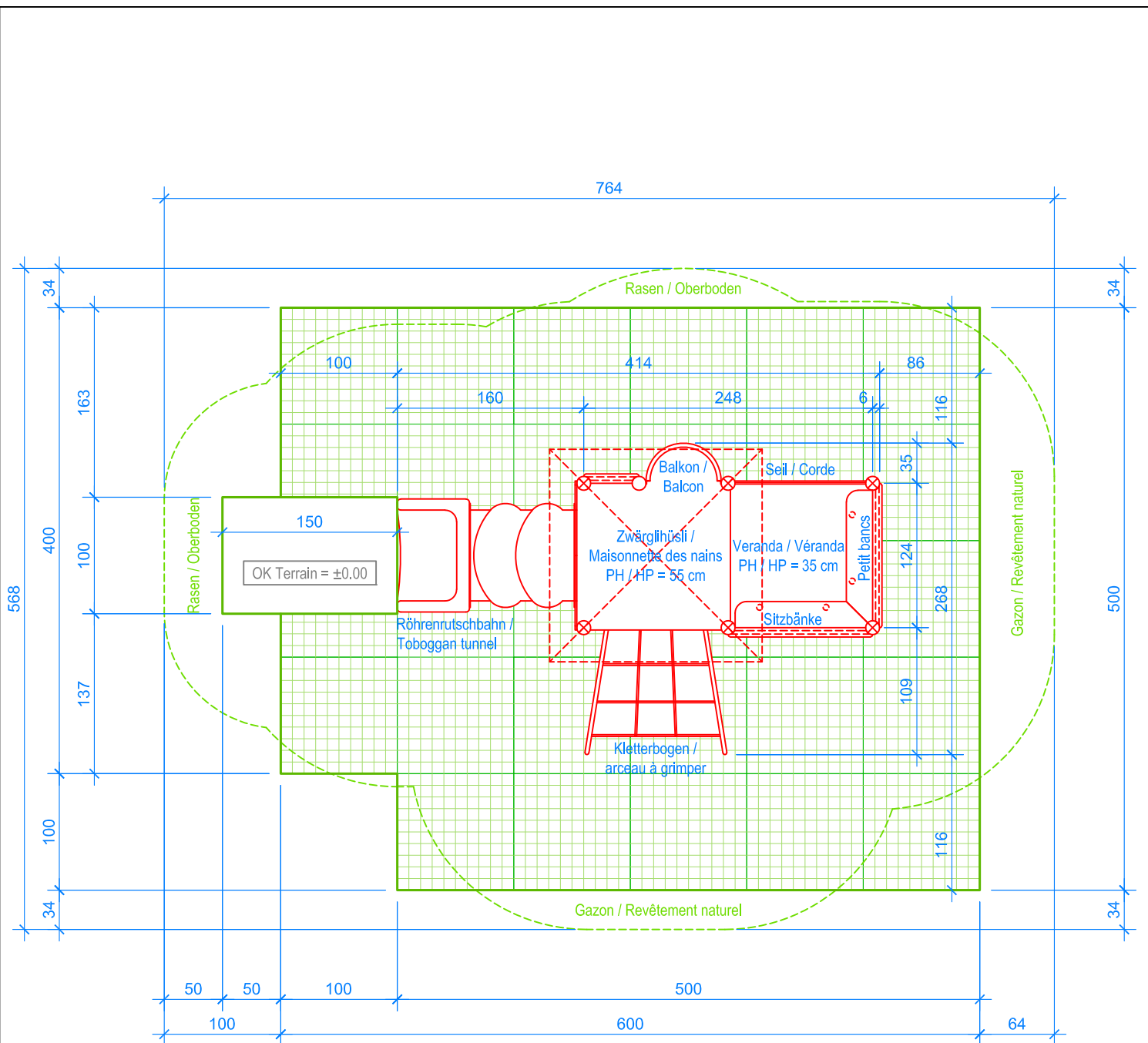
GRUNDRISS / PLAN 1:50
