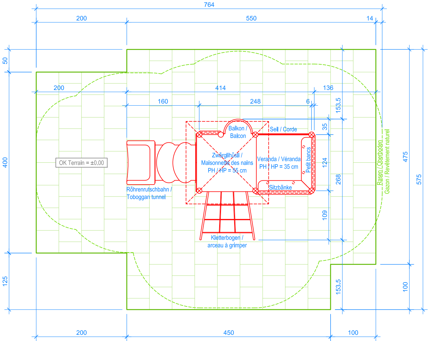
GRUNDRISS / PLAN 1:50
