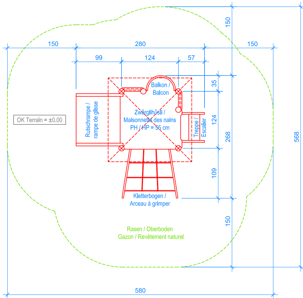
GRUNDRISS / PLAN 1:50
