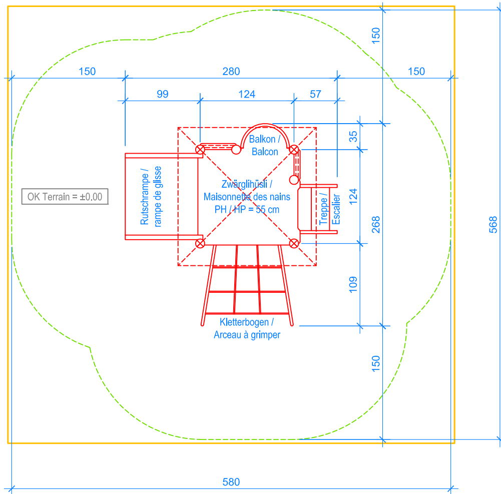
GRUNDRISS / PLAN 1:50
