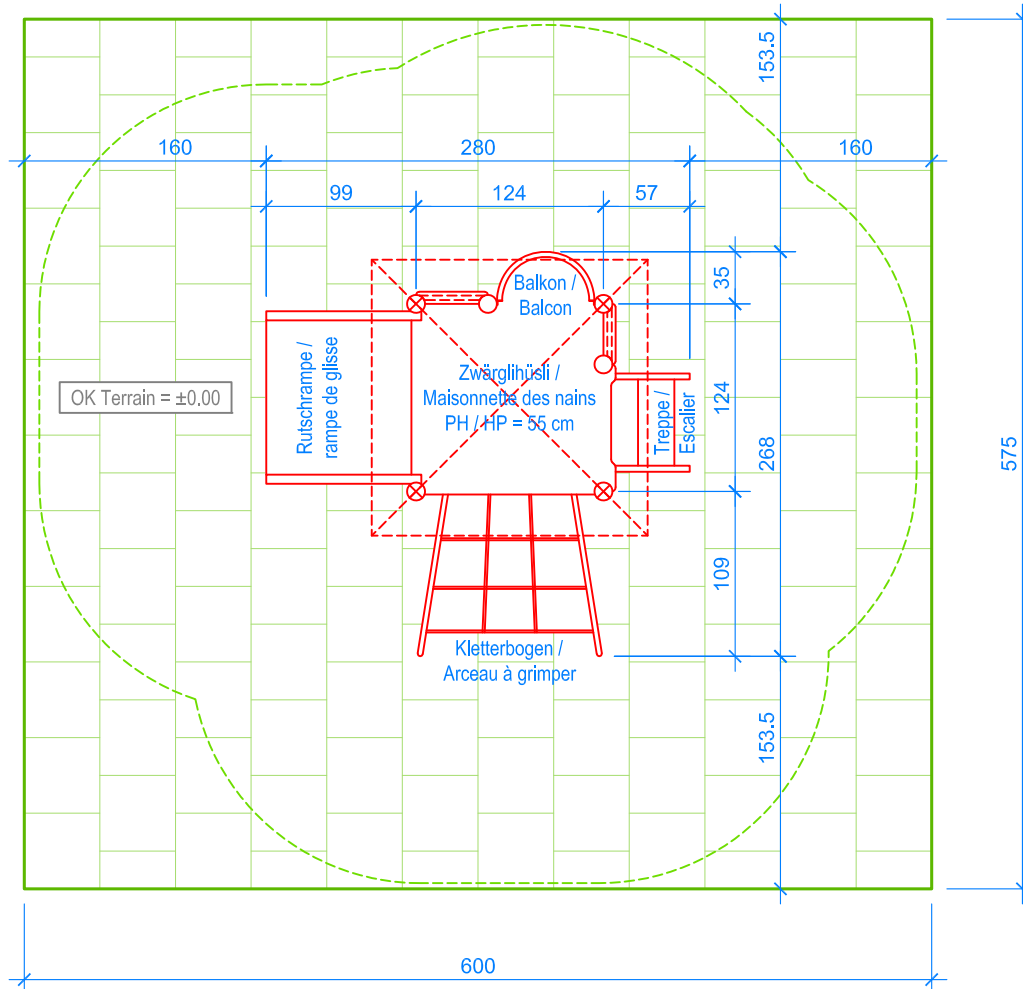
GRUNDRISS / PLAN 1:50
