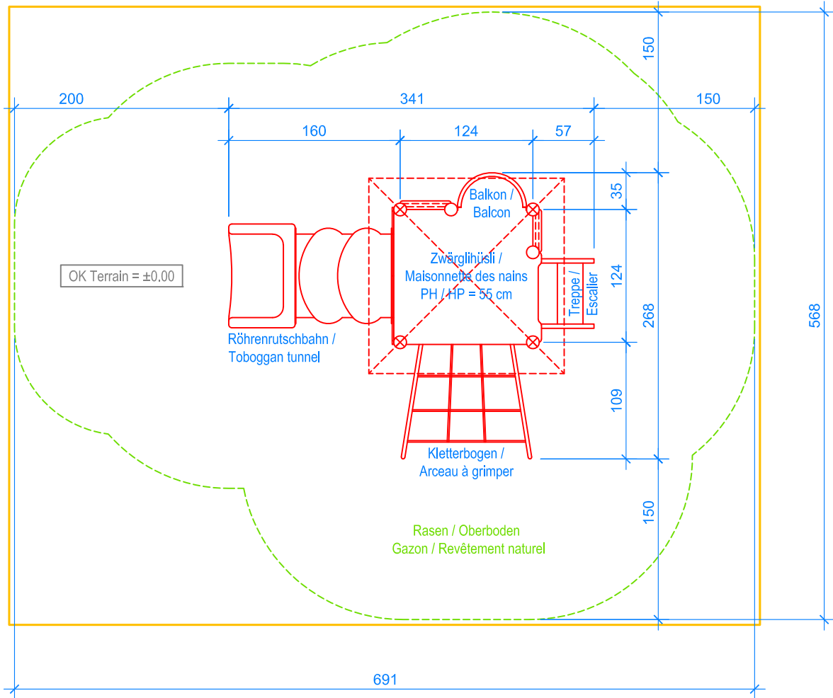
GRUNDRISS / PLAN 1:50
