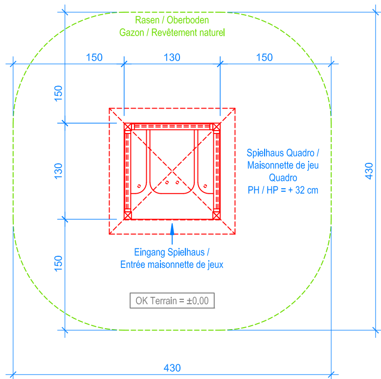
GRUNDRISS / PLAN 1:50
