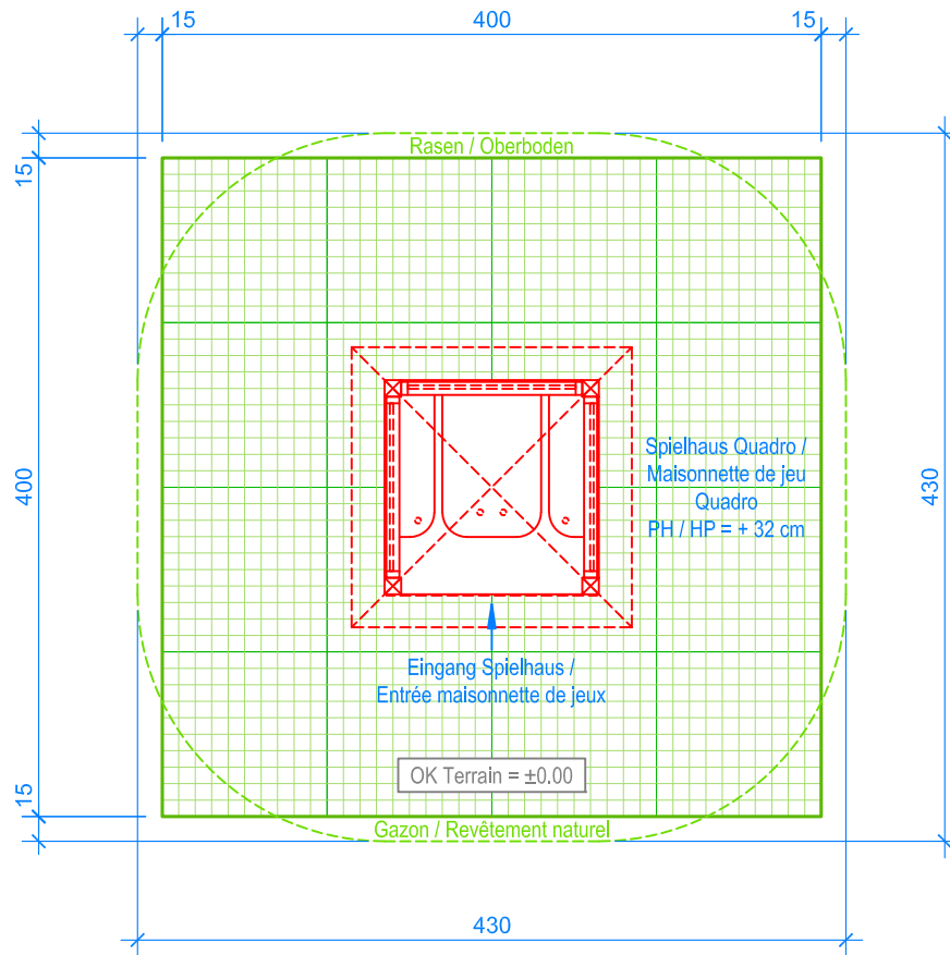
GRUNDRISS / PLAN 1:50
