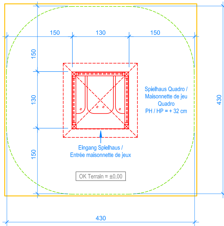
GRUNDRISS / PLAN 1:50
