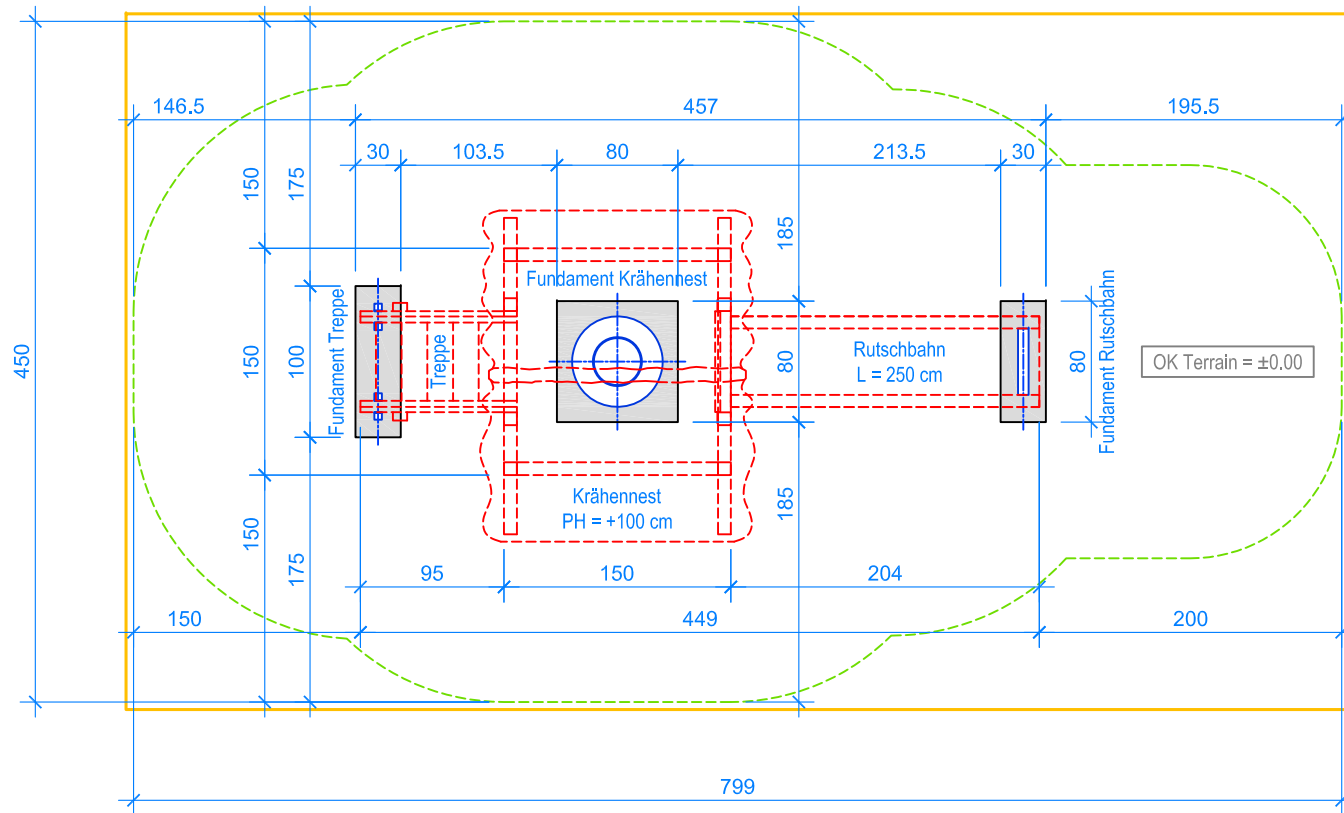
GRUNDRISS 1:50
