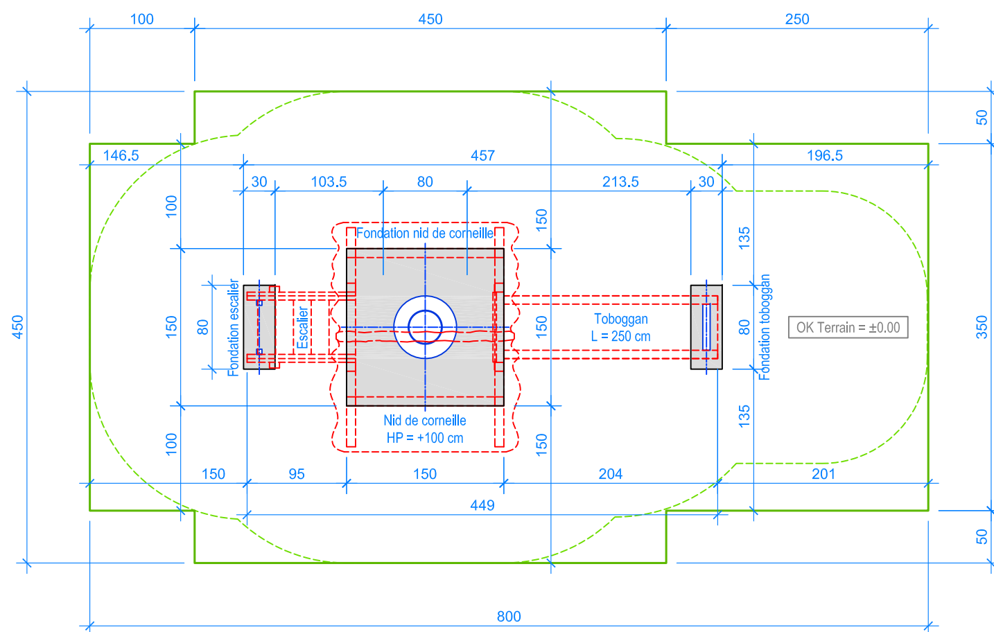
PLAN 1:50
