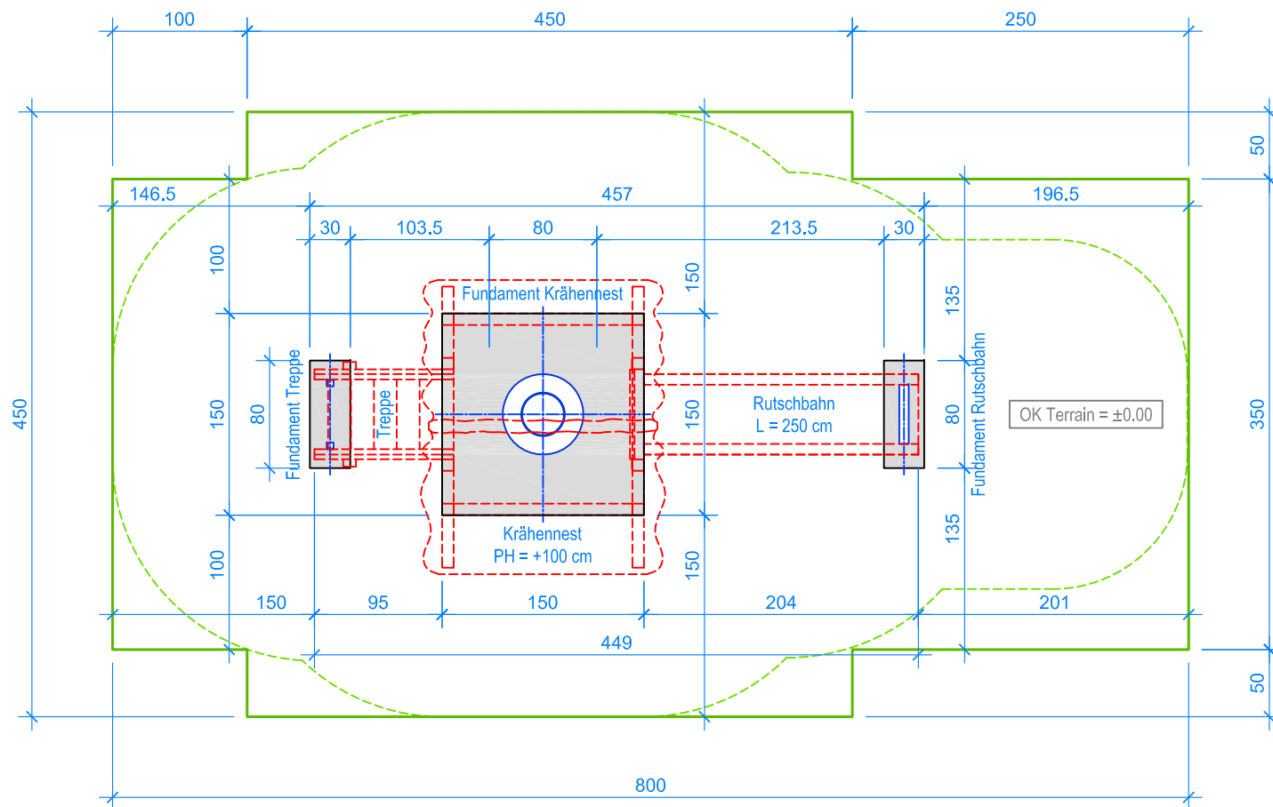
GRUNDRISS 1:50
