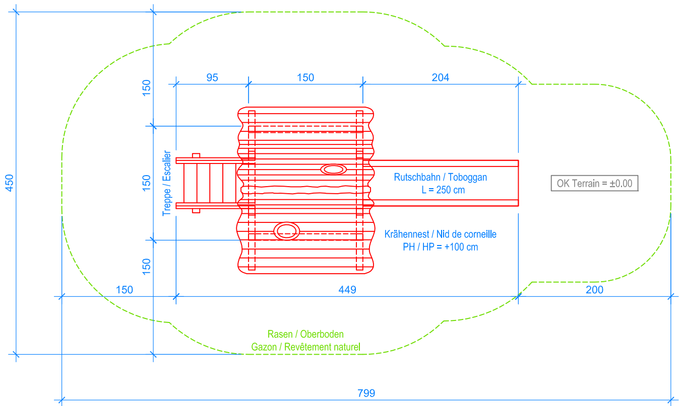
GRUNDRISS / PLAN 1:50
