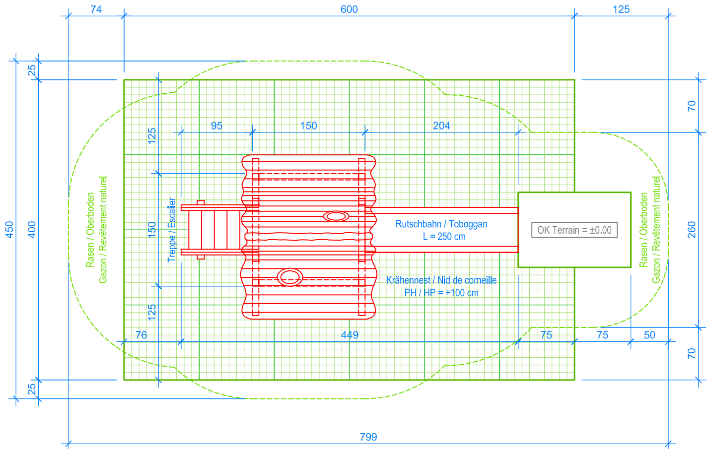
GRUNDRISS / PLAN 1:50
