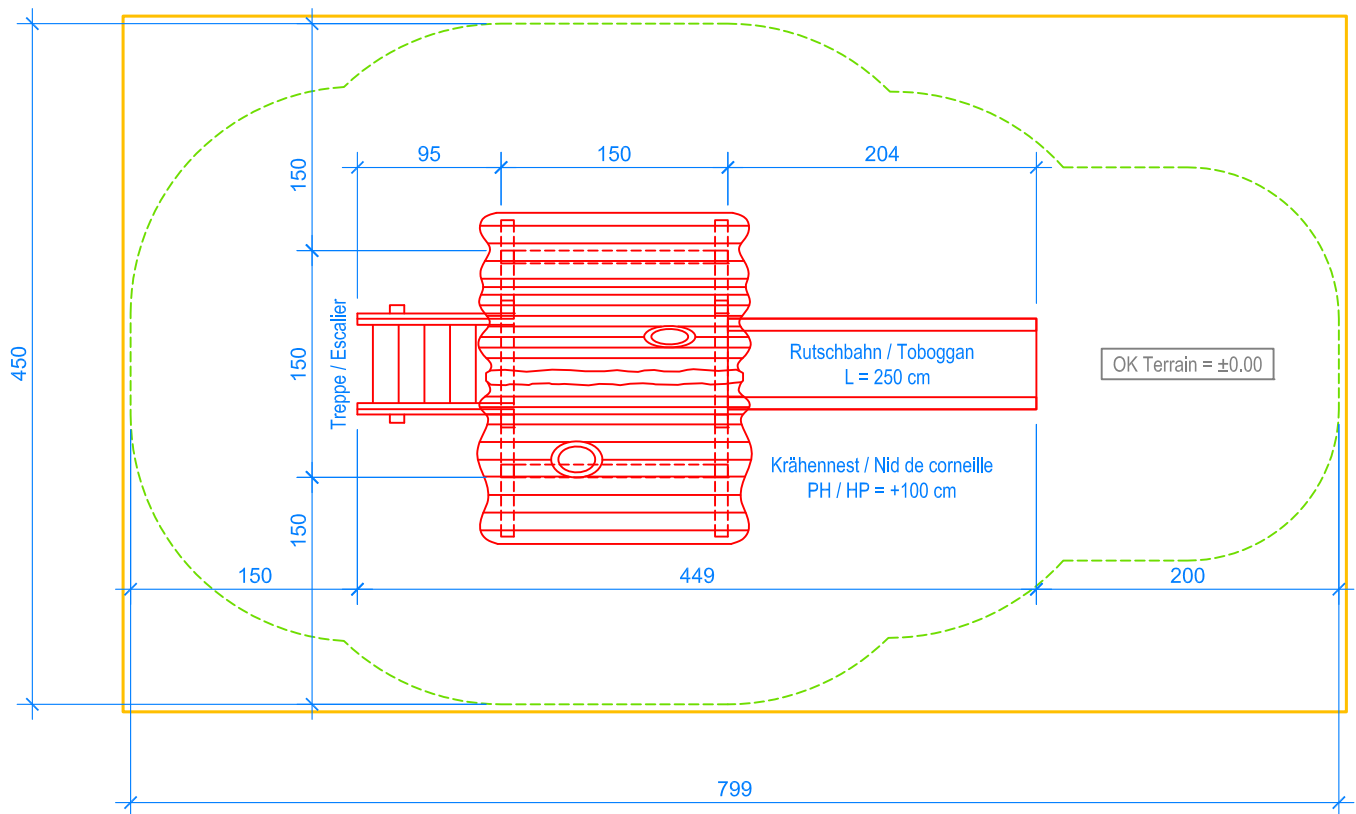
GRUNDRISS / PLAN 1:50
