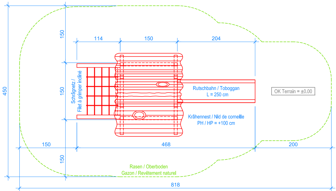
GRUNDRISS / PLAN 1:50
