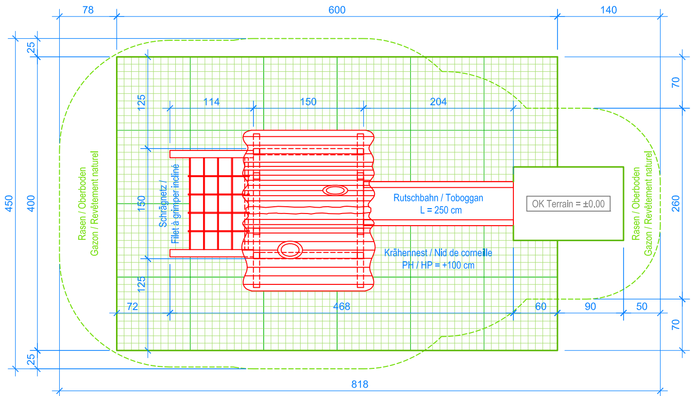
GRUNDRISS / PLAN 1:50
