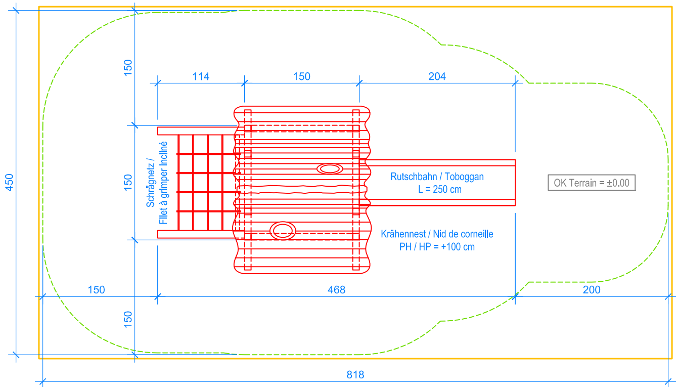
GRUNDRISS / PLAN 1:50
