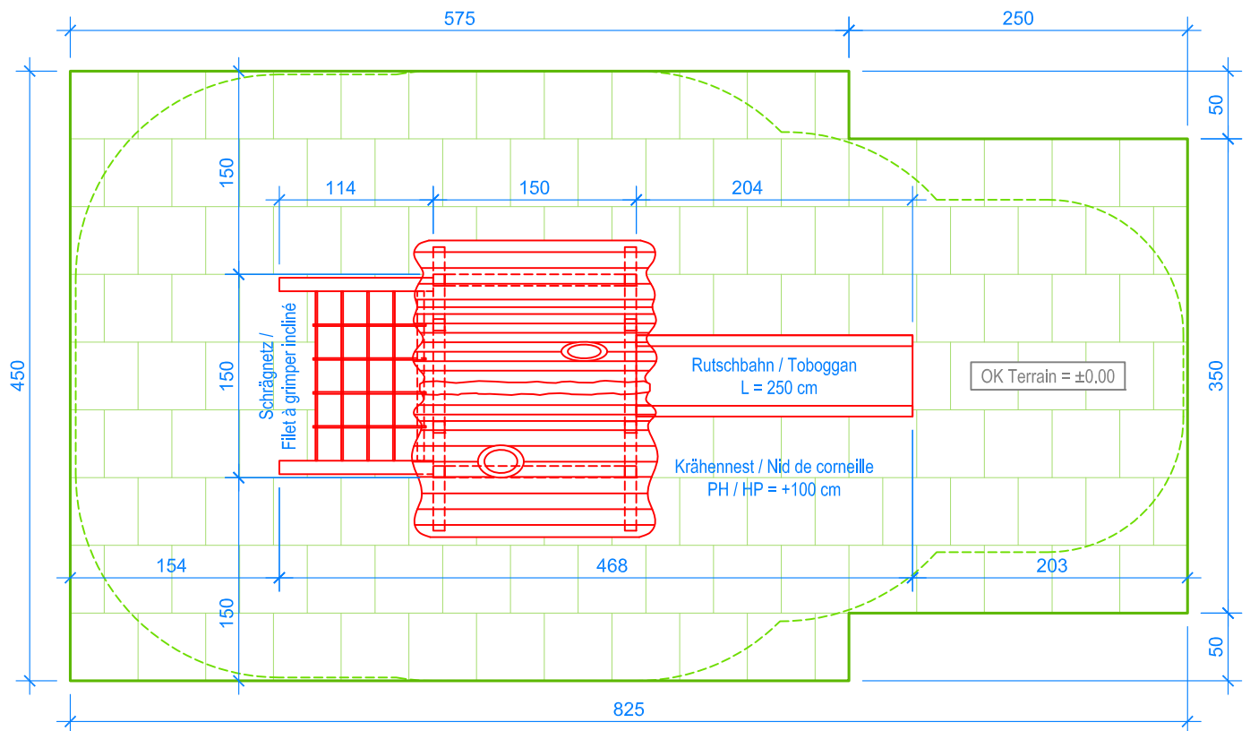
GRUNDRISS / PLAN 1:50
