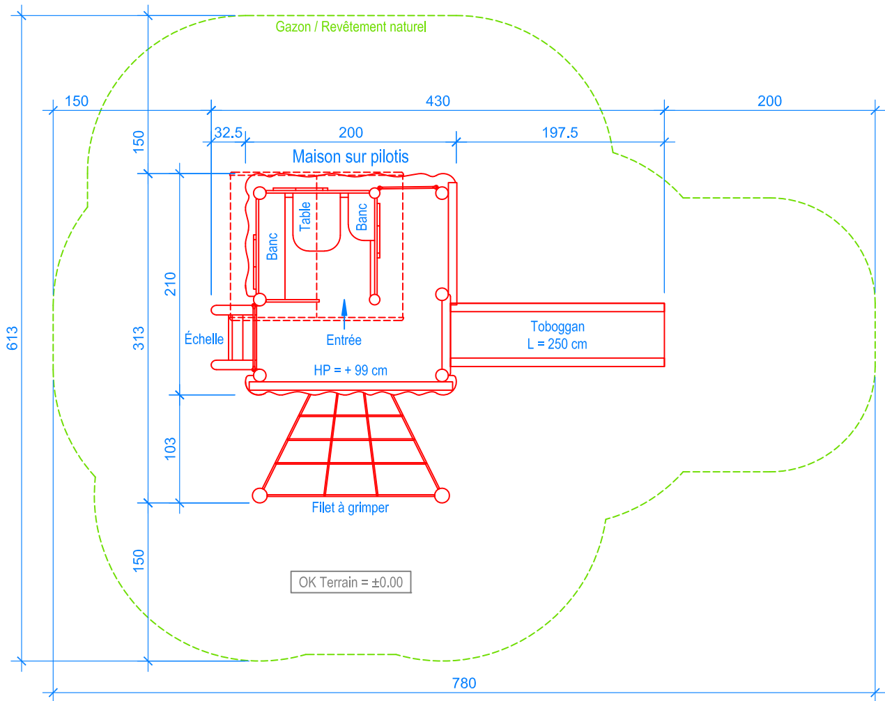
PLAN 1:50
