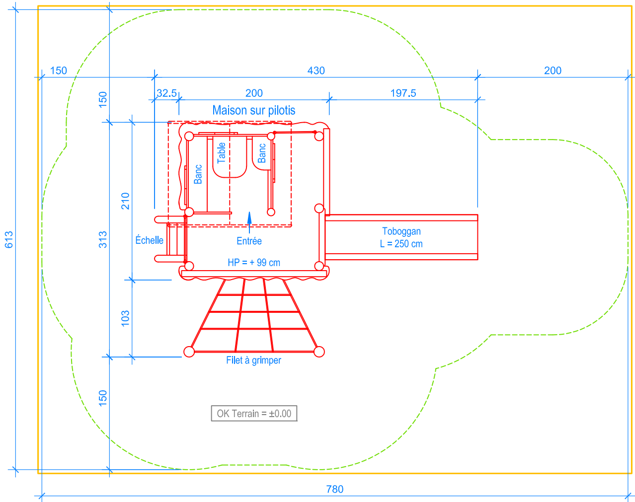
PLAN 1:50
