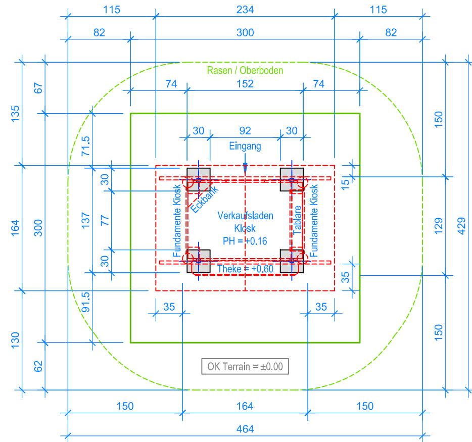
GRUNDRISS 1:50
