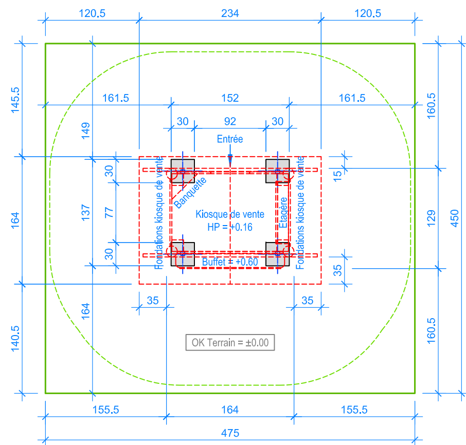
PLAN 1:50
