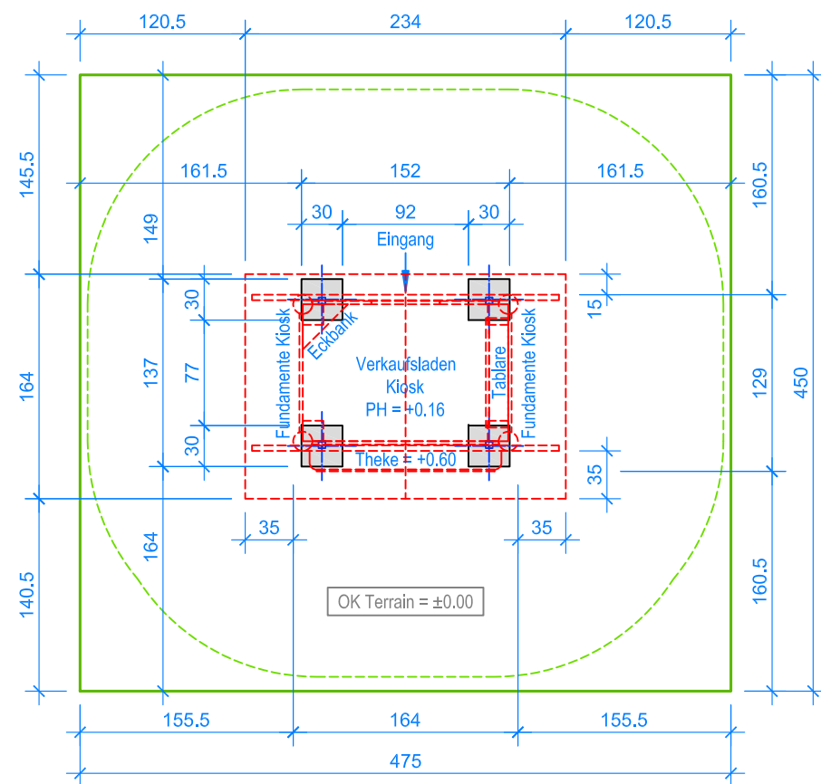
GRUNDRISS 1:50
