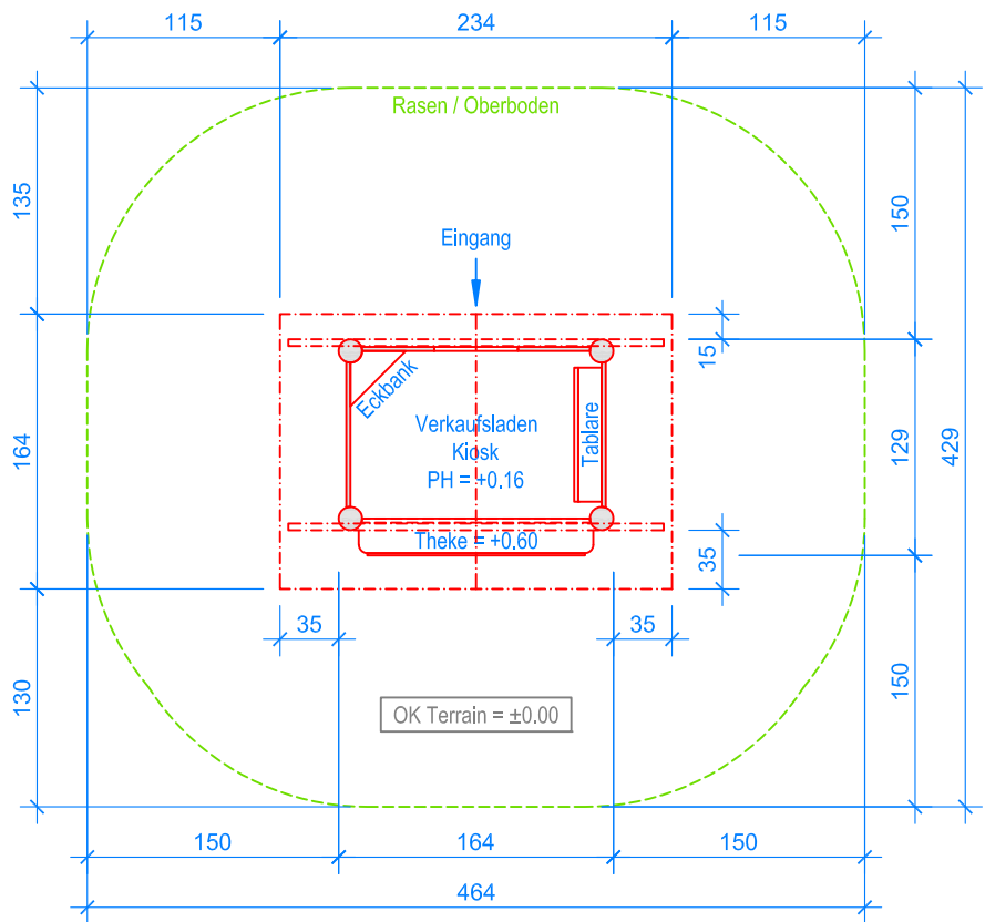
GRUNDRISS 1:50
