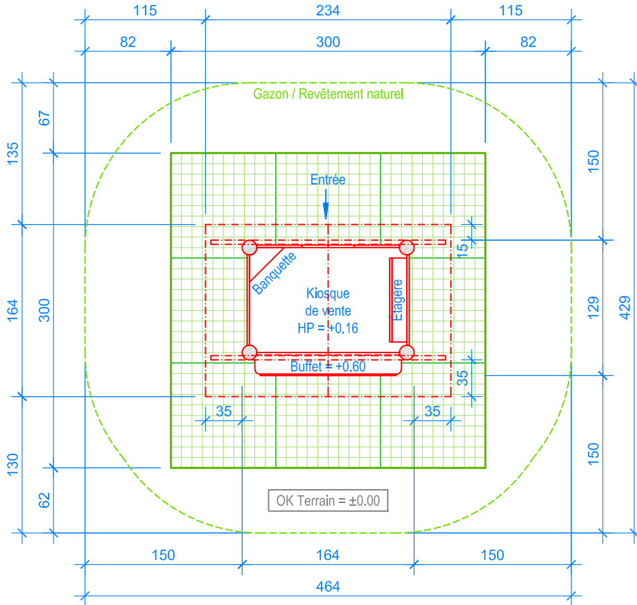
PLAN 1:50
