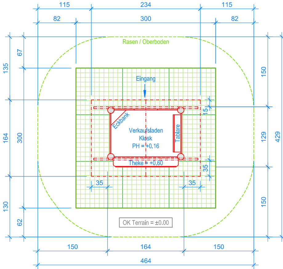
GRUNDRISS 1:50
