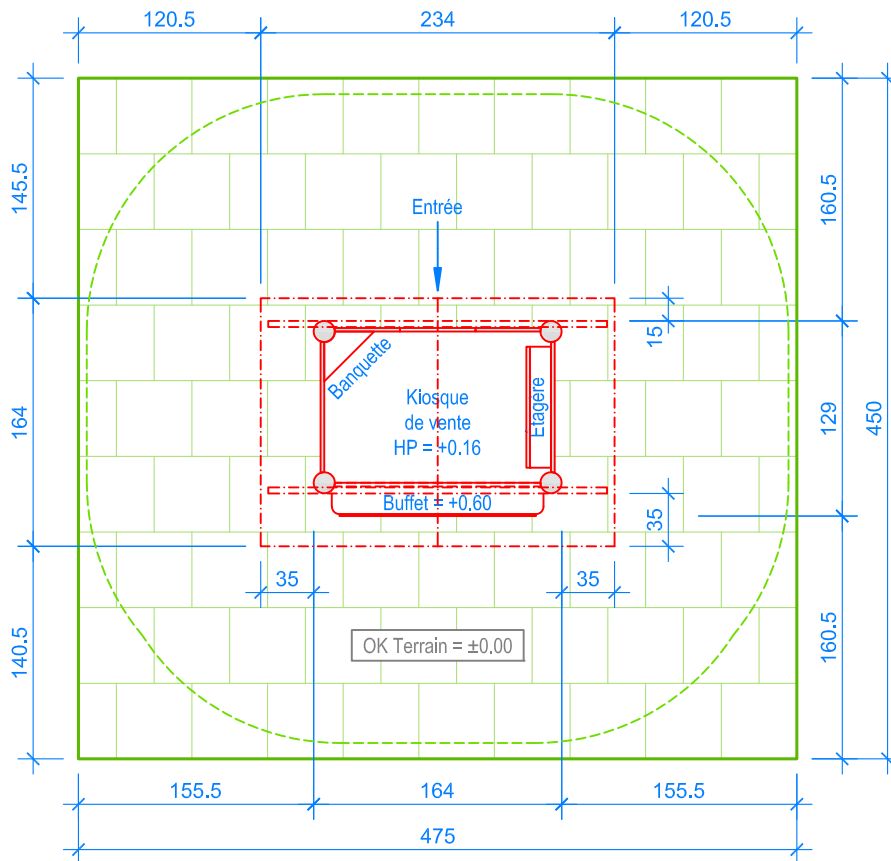
PLAN 1:50
