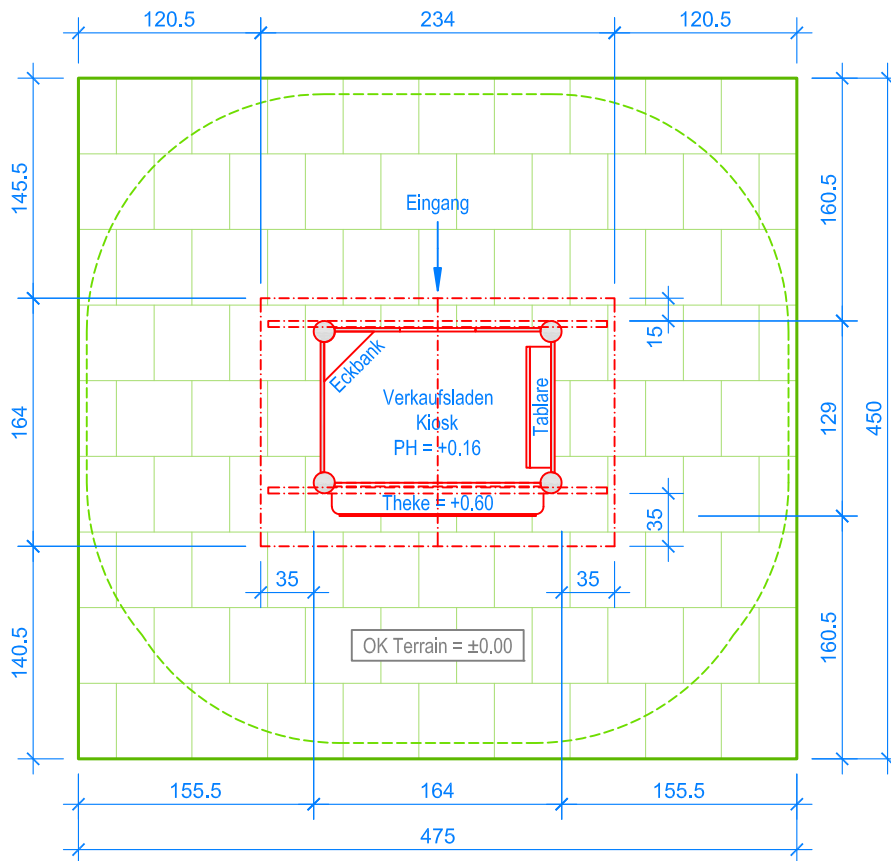
GRUNDRISS 1:50
