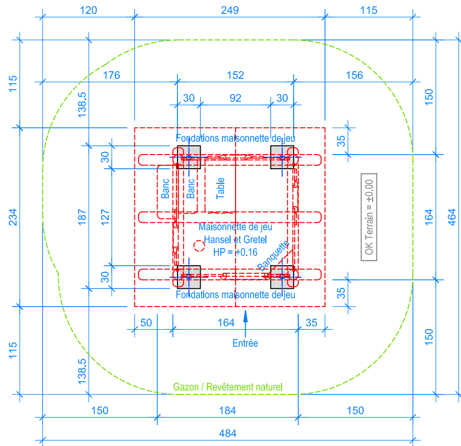
PLAN 1:50
