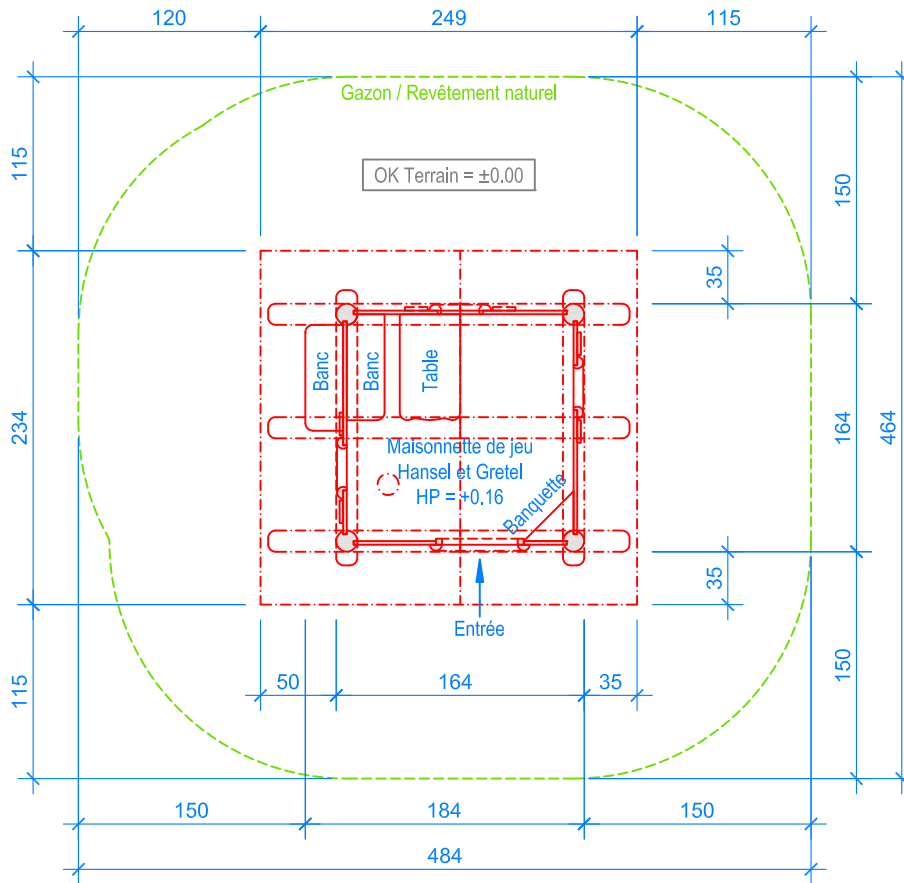
PLAN 1:50
