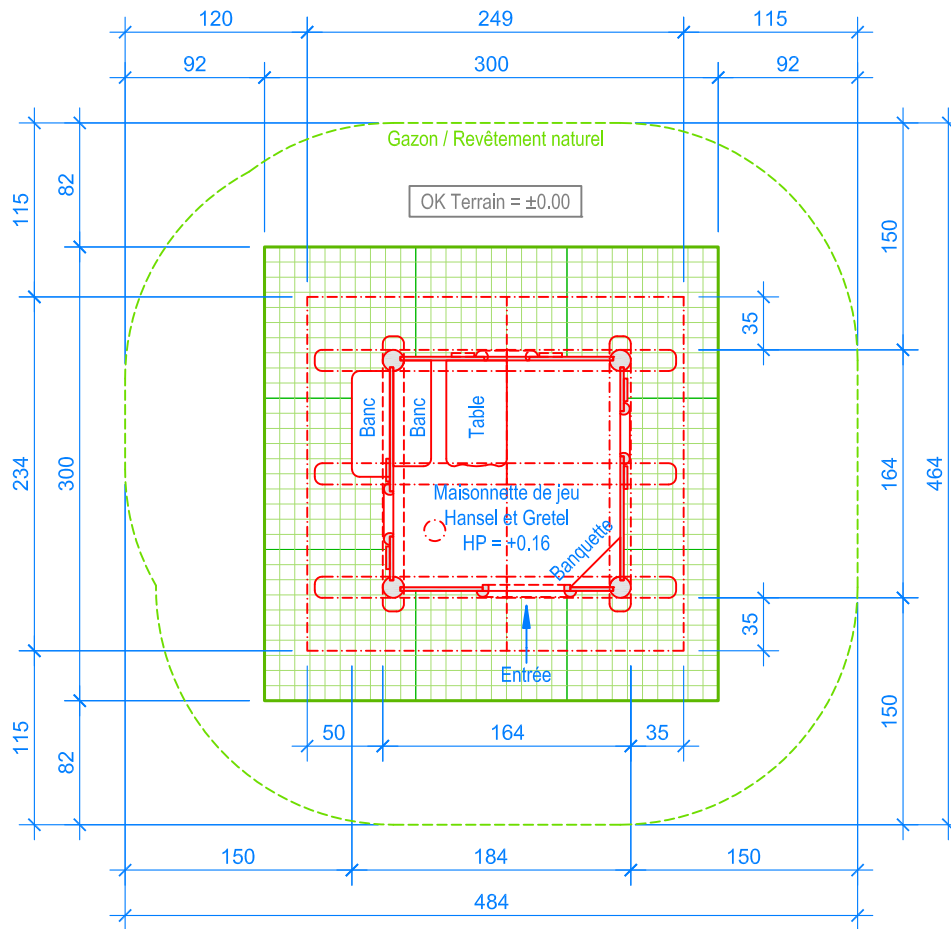
PLAN 1:50
