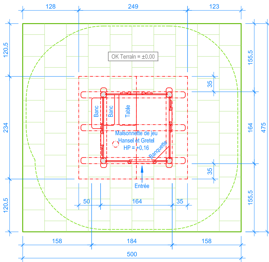
PLAN 1:50
