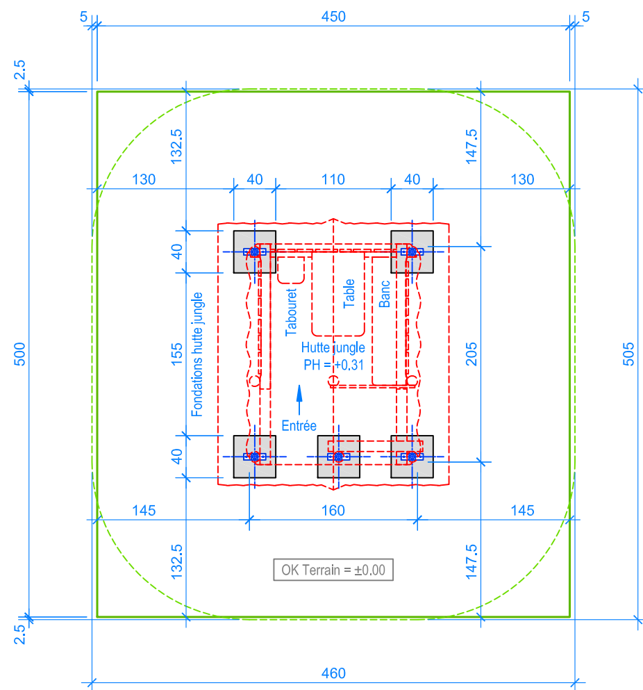
PLAN 1:50
