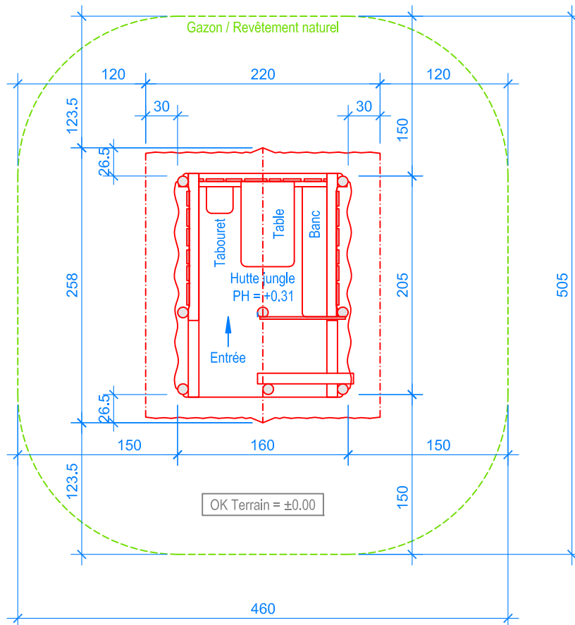
PLAN 1:50
