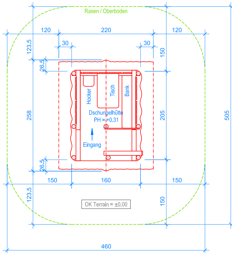
GRUNDRISS 1:50
