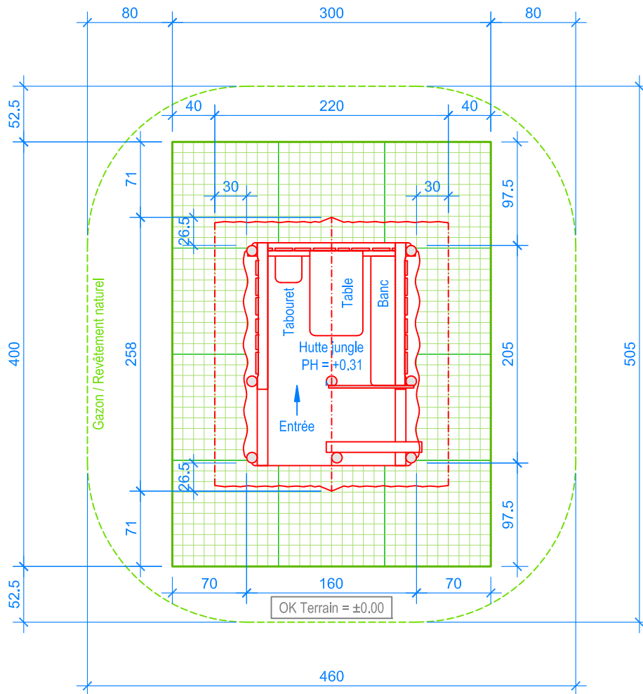
PLAN 1:50
