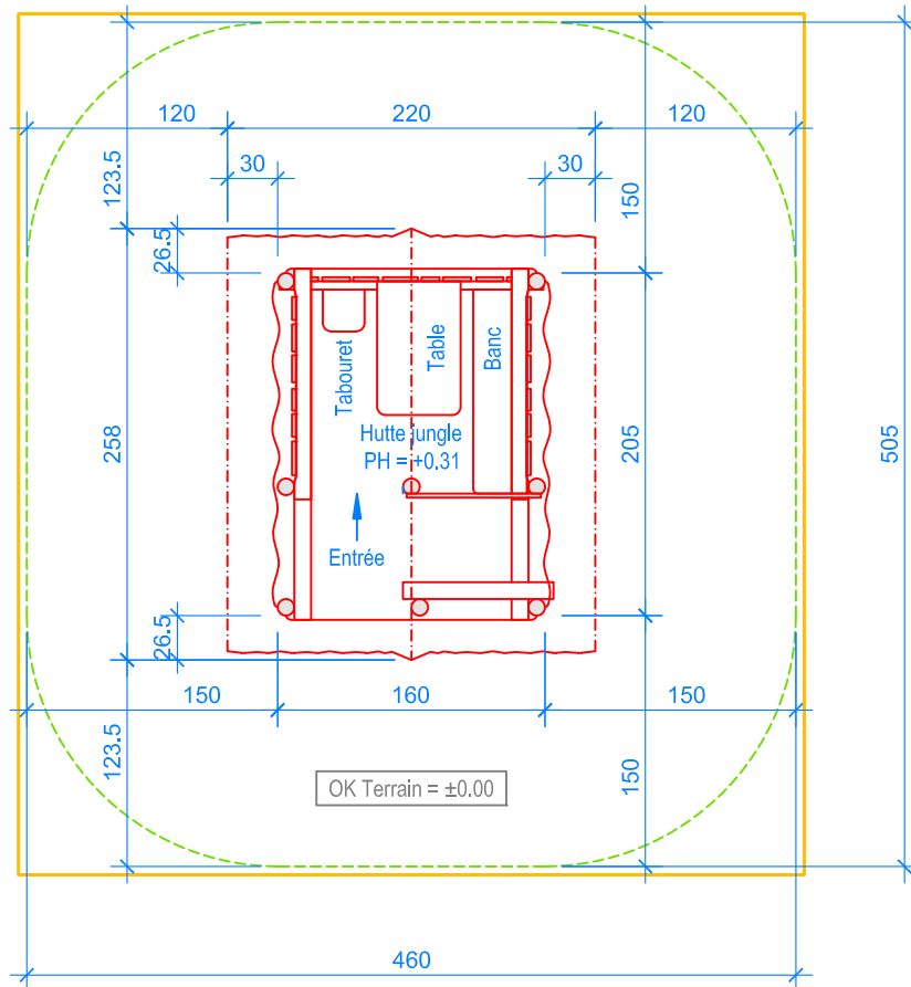
PLAN 1:50
