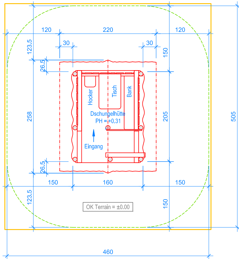
GRUNDRISS 1:50
