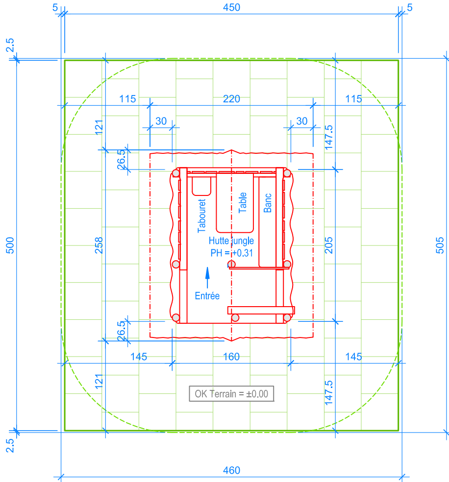
PLAN 1:50
