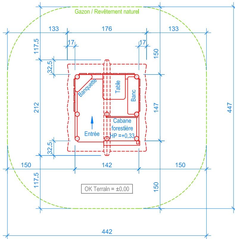
PLAN 1:50
