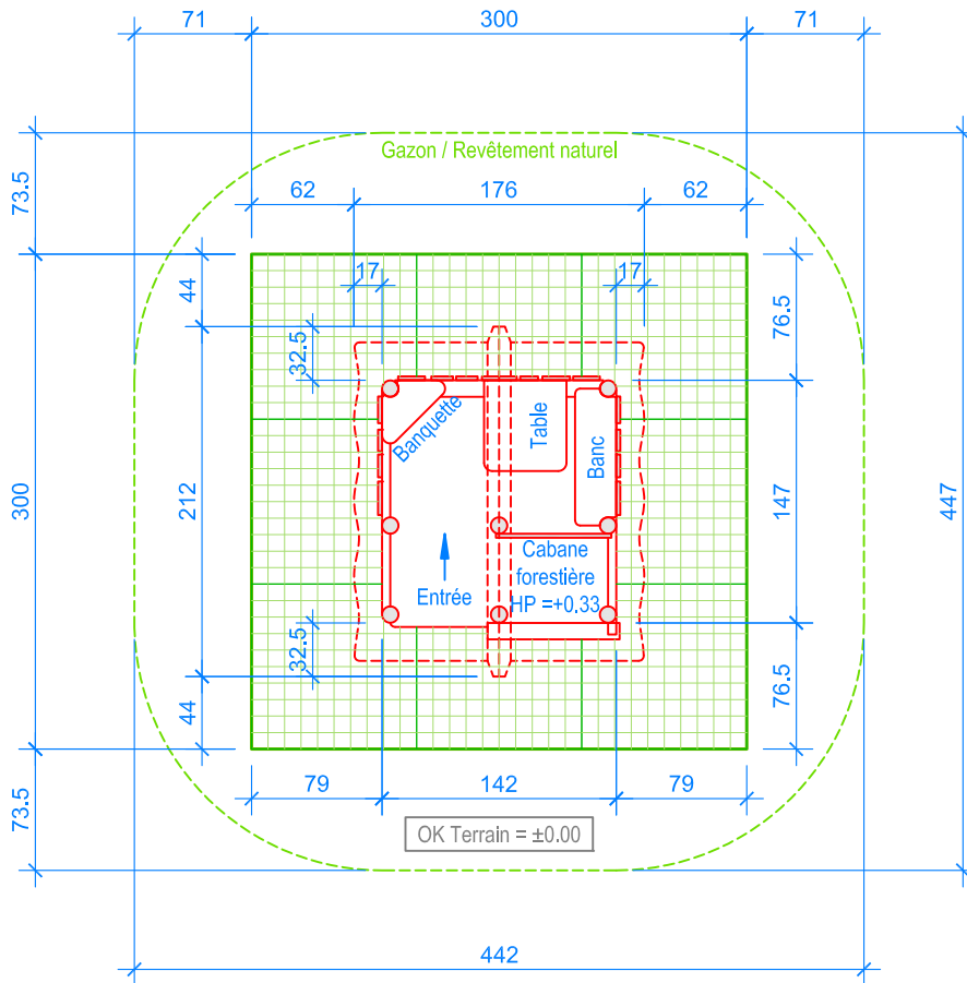
PLAN 1:50
