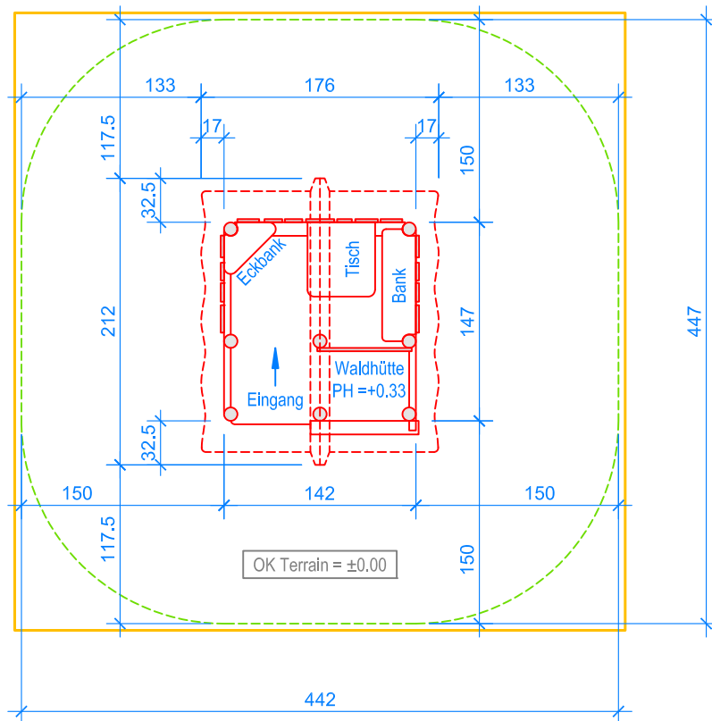
GRUNDRISS 1:50
