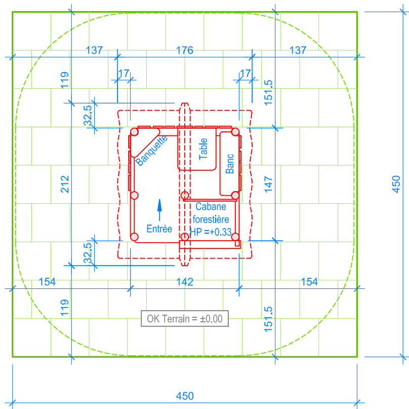
PLAN 1:50
