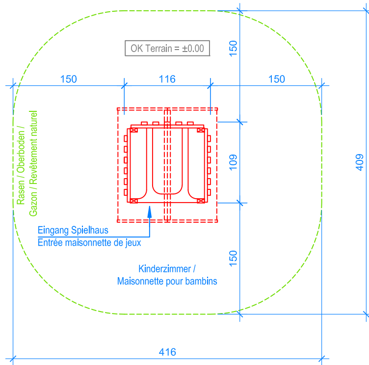
GRUNDRISS / PLAN 1:50
