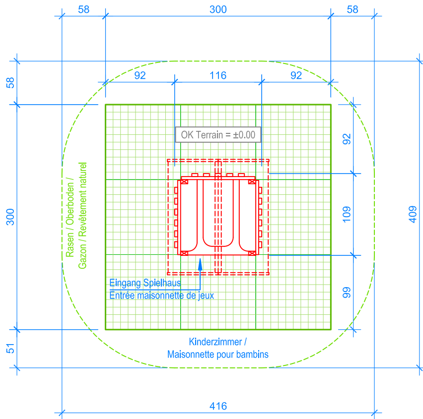
GRUNDRISS / PLAN 1:50
