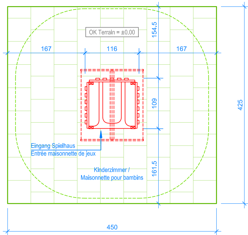
GRUNDRISS / PLAN 1:50
