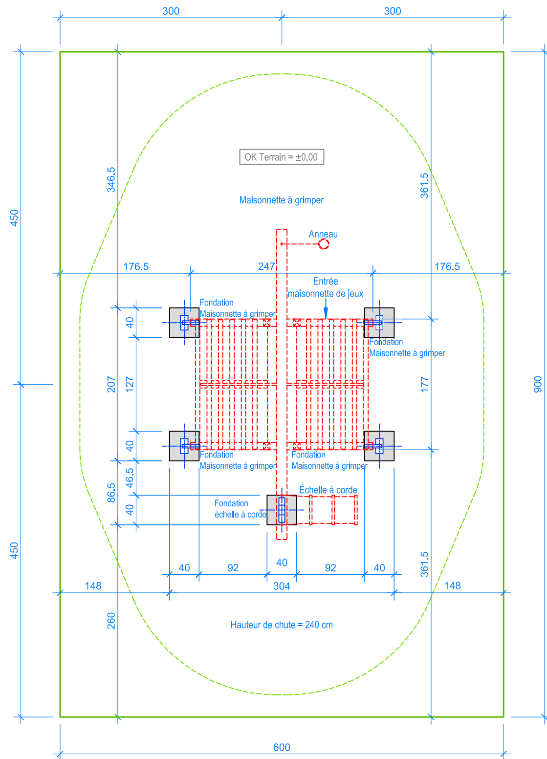
PLAN 1:50
