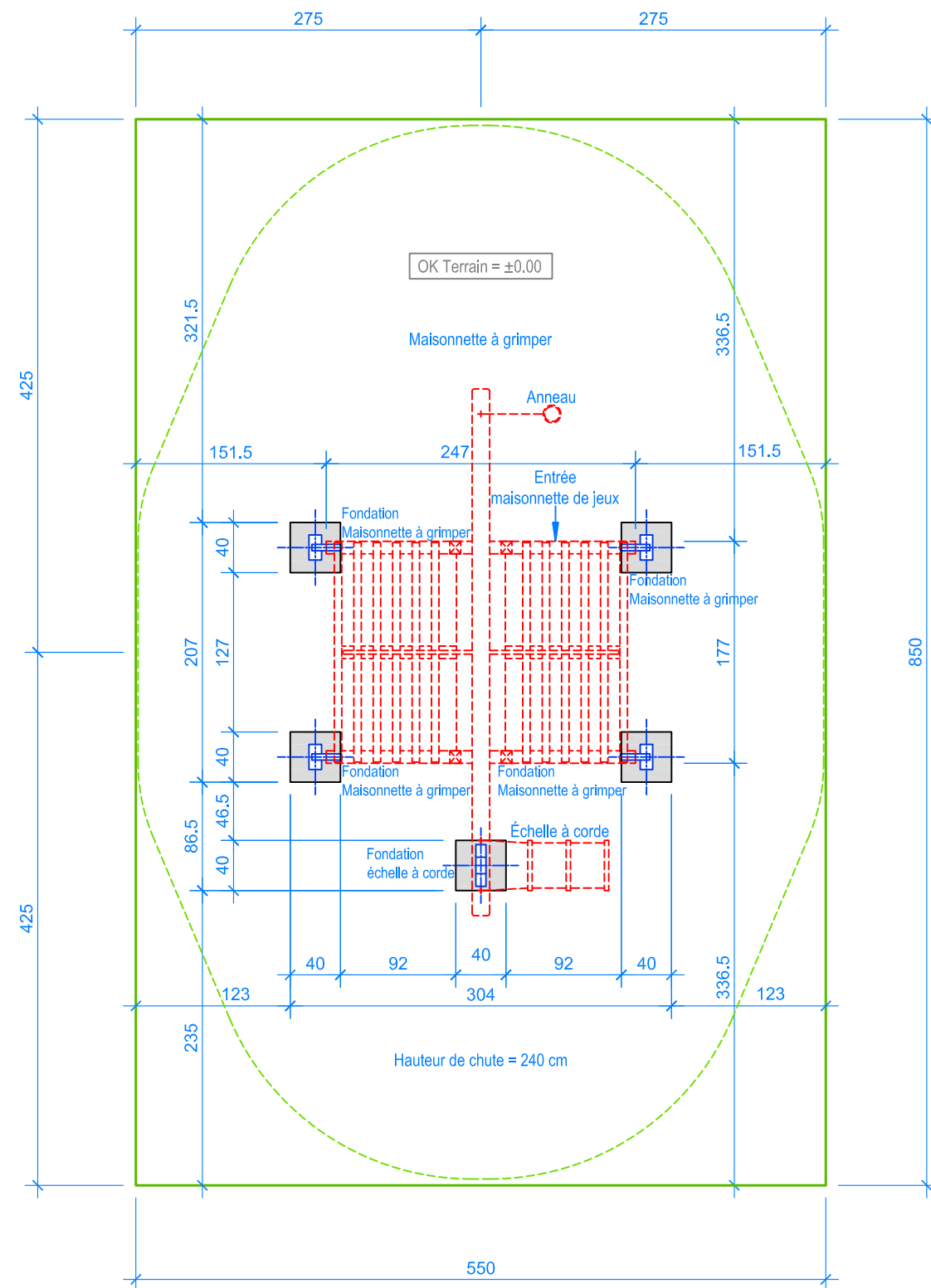
PLAN 1:50
