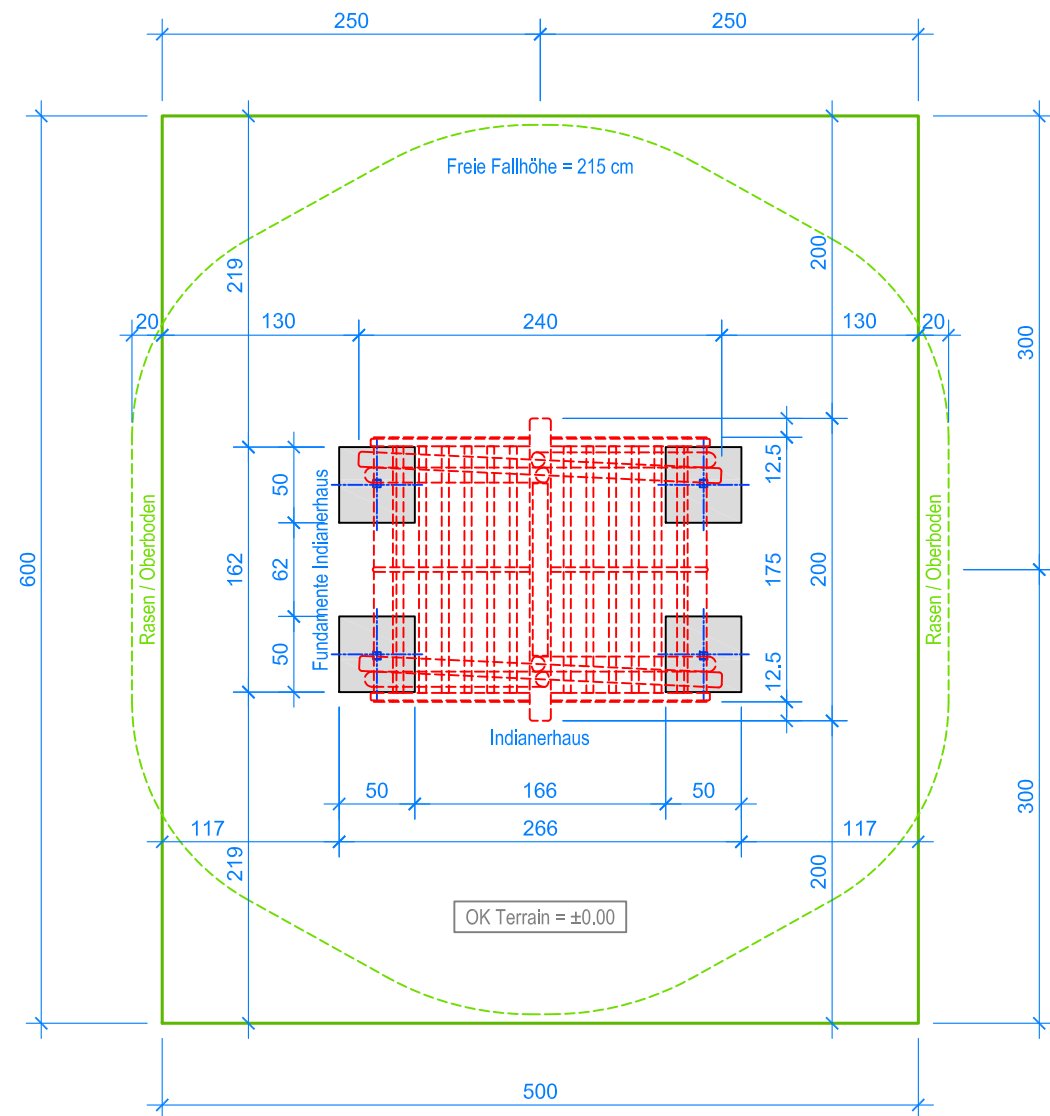
GRUNDRISS 1:50
